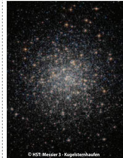
© HST: Messier 3 - Kugelsternhaufen
